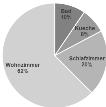
Abbildung 4: Verteilung der SHT-Heizleistungen (Ventilöffnungen) nach Raumtypen aller Wohnungen (n=14)
