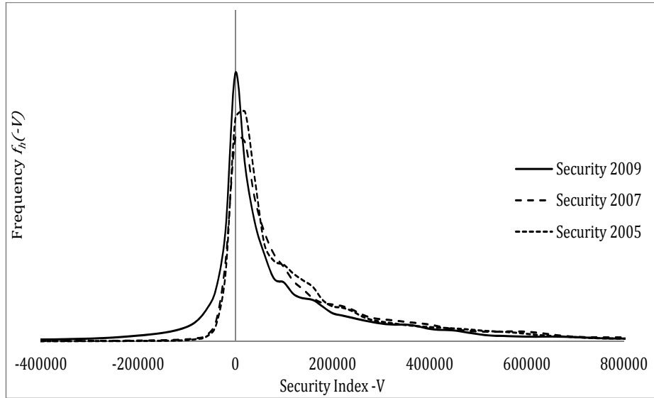
Panel A: USA \gamma = 1
